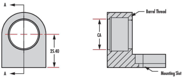
L-Slot Type (#36-410 & #36-416)
