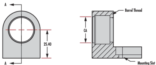
L-Slot Type (#36-410 & #36-416)
